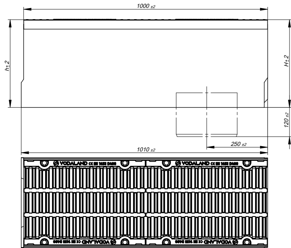
Лоток з решіткою щілинною D400
